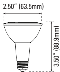
PAR20 3.68-oz
