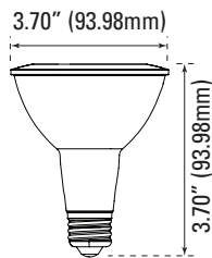
PAR30 6.56-oz
